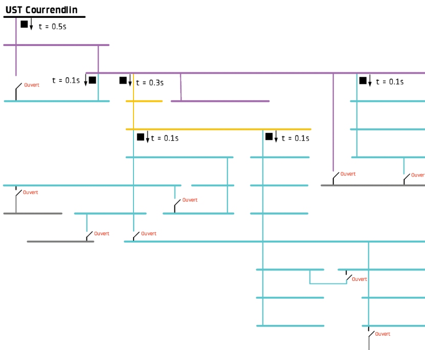
Selektivitätszonen des Erdschlussschutzes
