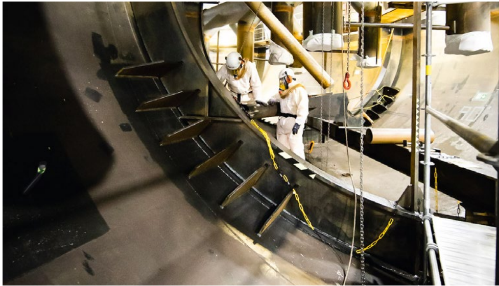
Demontagearbeiten im Torus. Foto: KKM
