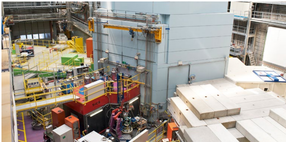
Spallations- neutronenquelle. Foto: PSI
