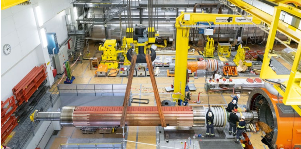
Generatorrevision: Beim Ziehen des Rotors ist Finger- spitzengefühl gefragt. Foto: KKG
