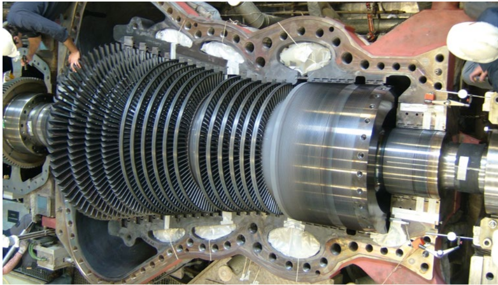
Inspektion der Hochdruckturbine. Foto: KKB
