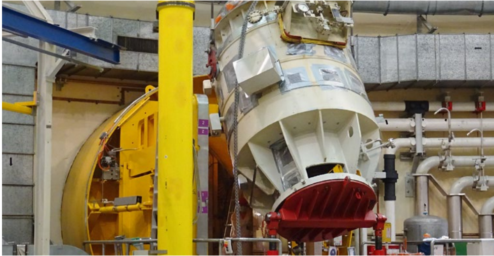
Austausch des Motors der Reaktor- hauptpumpe. Foto: KKB
